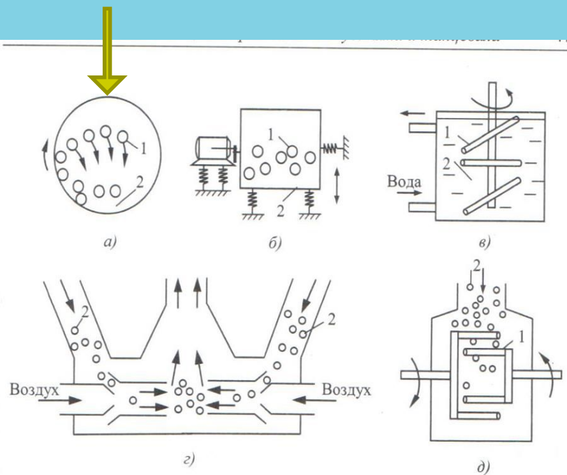
Рис. 4.3. Принципиальная схема мельниц для получения НЧ диспергированием: а – шаровая мельница, б – вибромельница, в – с вращающимися «пальцами», г – струйная мельница, д – с вращающимися навстречу «пальцами». 1 – шары, или «пальцы»; 2 – исходный материал, подвергающийся диспергированию.
