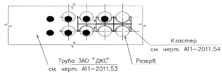
Разрез 1-1
