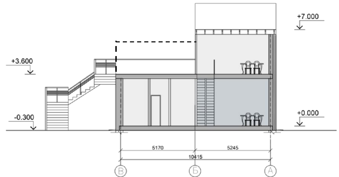
Разрез Б-Б, М1:100
