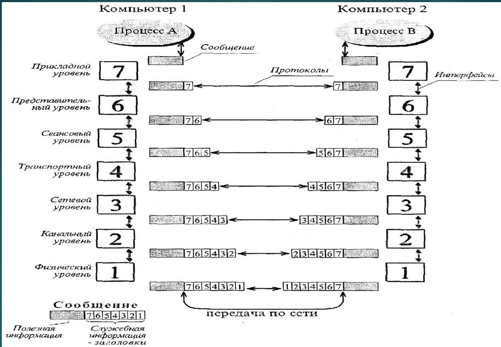
OSI ашық жүйелерінің өзара әрекеттесу үлгісі.
