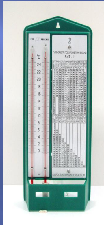
ПСИХОМЕТР
