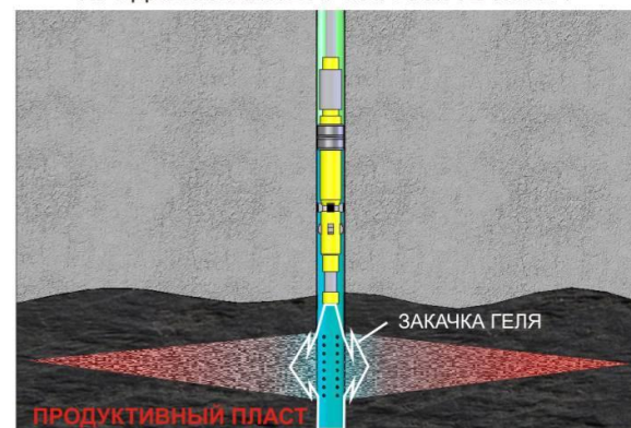
ПРОДАВЛИВАНИЕ ПРОПАНТА В ПЛАСТ
