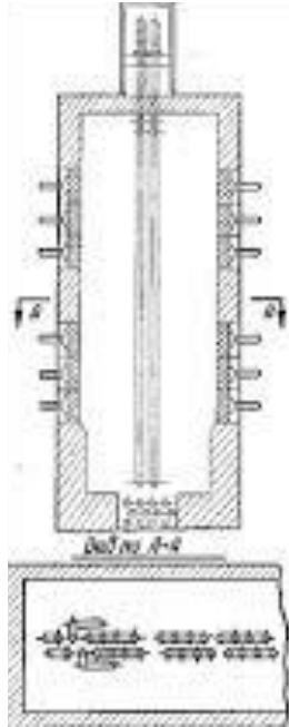
Печь с вертикальным змеевиком конструкции Гипрокаучук
