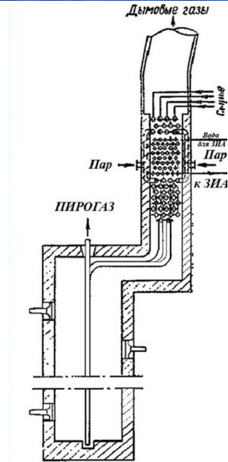
Печь фирмы Lummus типа SRT-I
