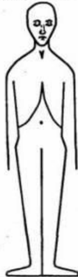
ЛЕПТОСОМАТИК
