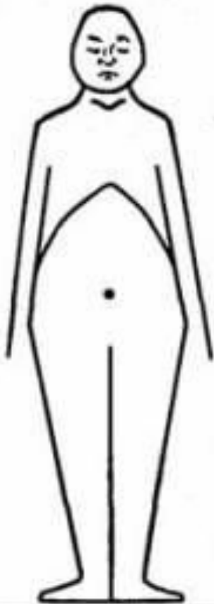
ДИСПЛАСТИК
