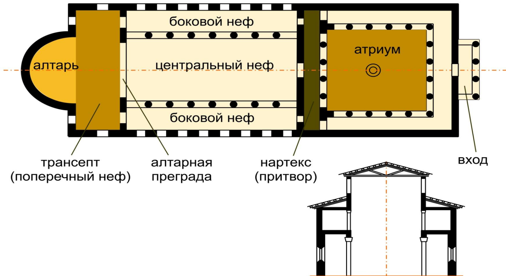
План и конструкция христианской базилики
