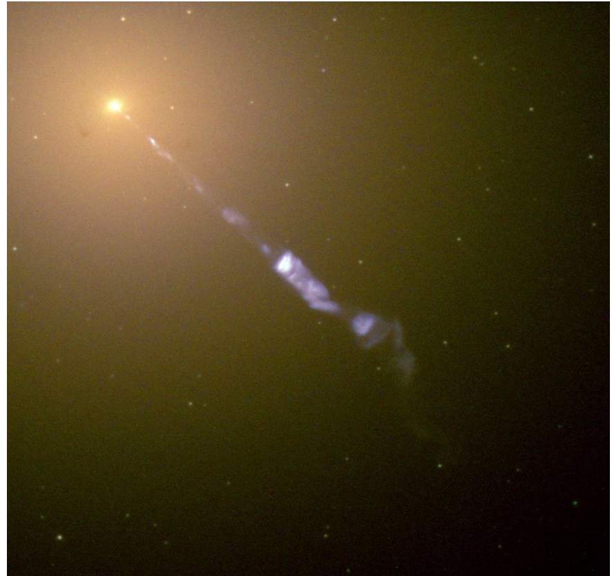
Галактика M87
