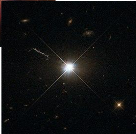
Квазар C273
