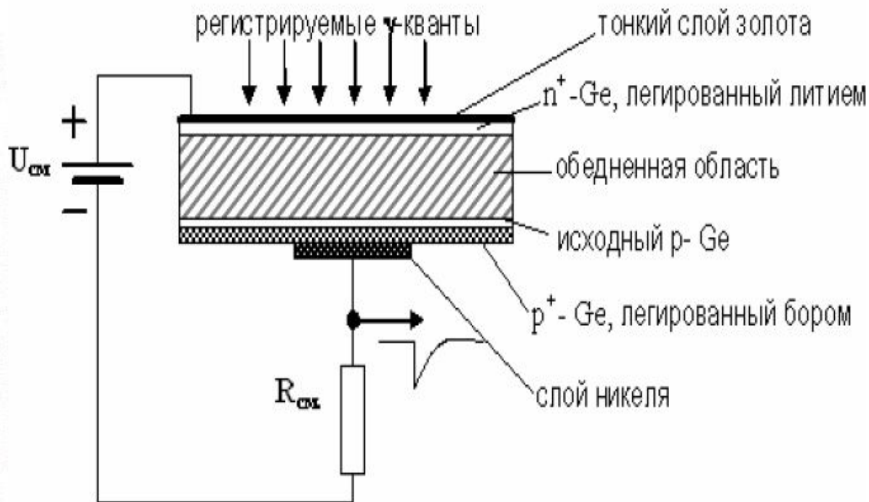
Рис. 2 Структура HPGe-детектора
