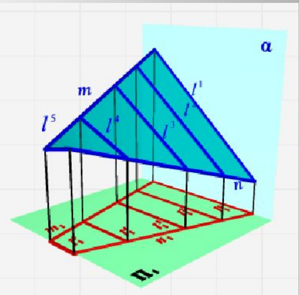
Гиперболический
