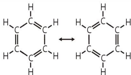
Benzol Kekulé-Strukturformel (Mesomerie)
