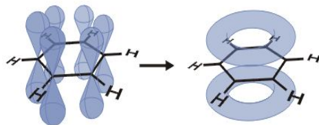
Benzol 6 p_z -Orbitale
