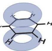
Benzol delokalisierte \pi -Orbitalwolke
