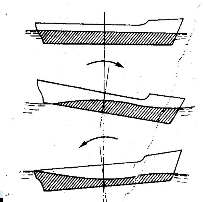
Килевая качка
