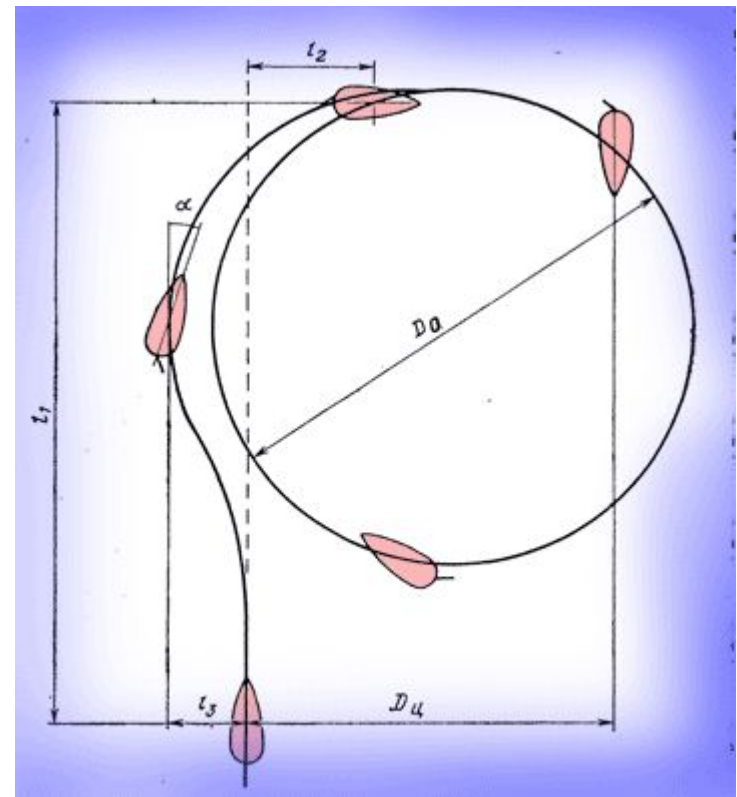
Элементы циркуляции
