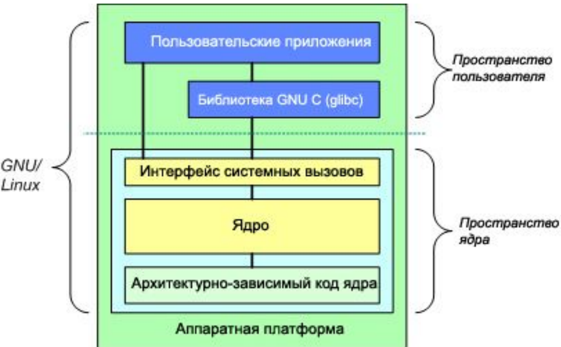
Структура ОС Linux
