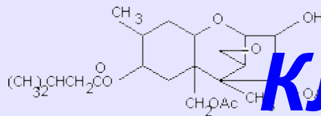
T-2 токсин
