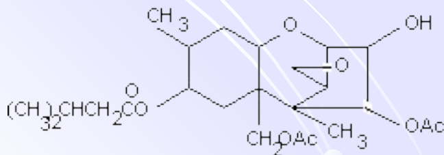
T-2 токсин
