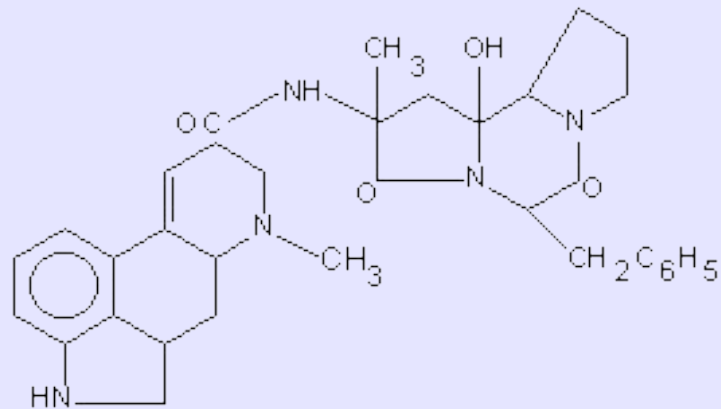
эрготамин
