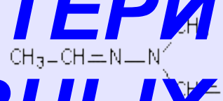
гиромитрин
