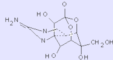
тетродотоксин рыбы
