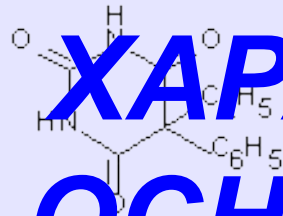
фенobarбитал
