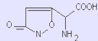
иботеновая кислота
