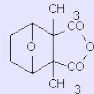
кантаридин жуки
