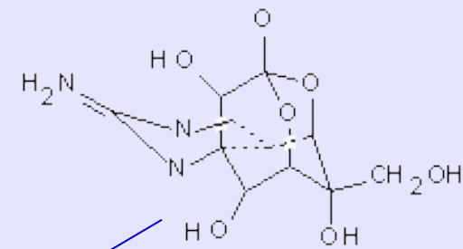
тетродотоксин рыбы
