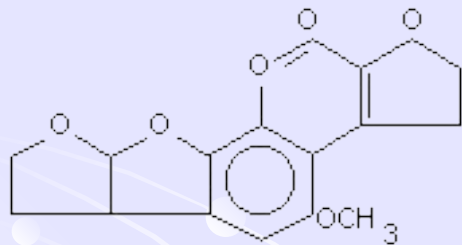
афлатоксин В 1
