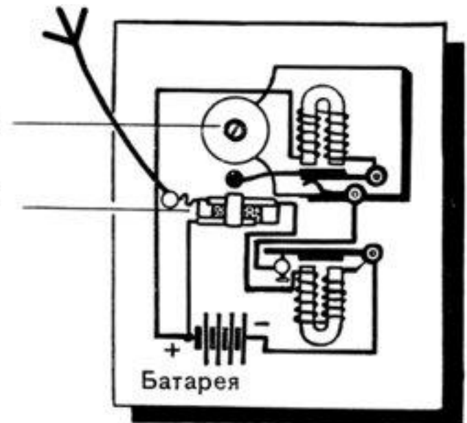
Рис. 2 Эскизный чертёж приемника
